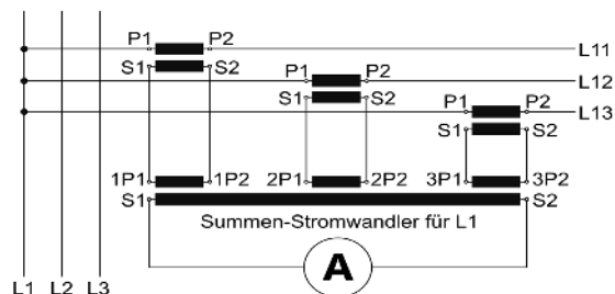
Anschlussbild
